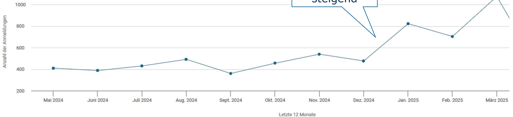
Benutzer-Anmeldungen
